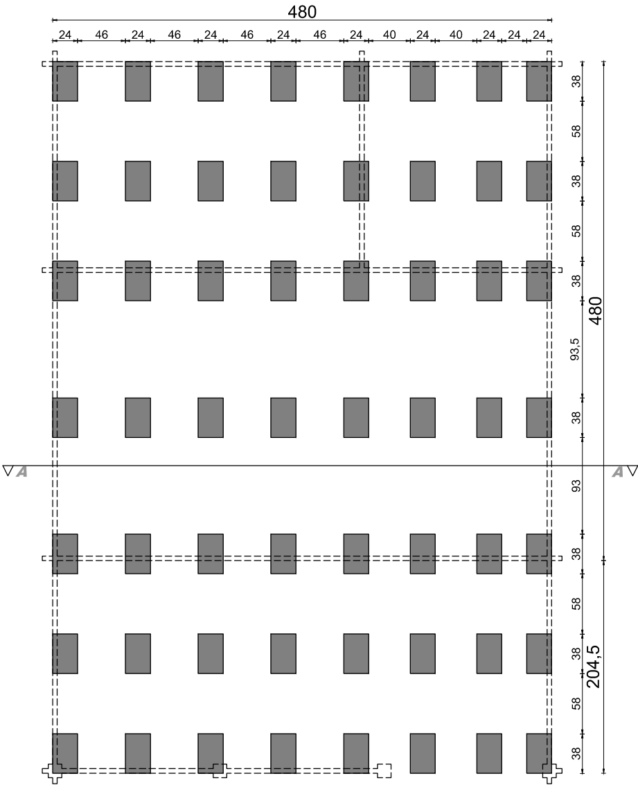
rzut fundamentów
