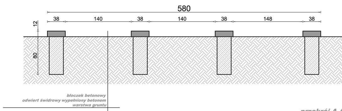
przekrój A-A
