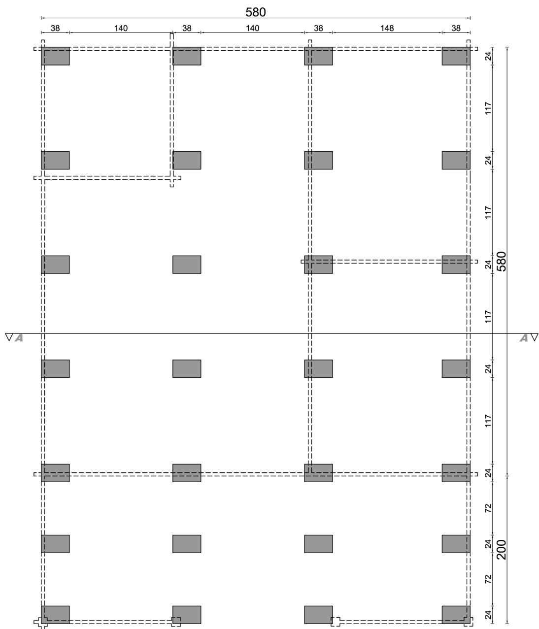
rzut fundamentów
