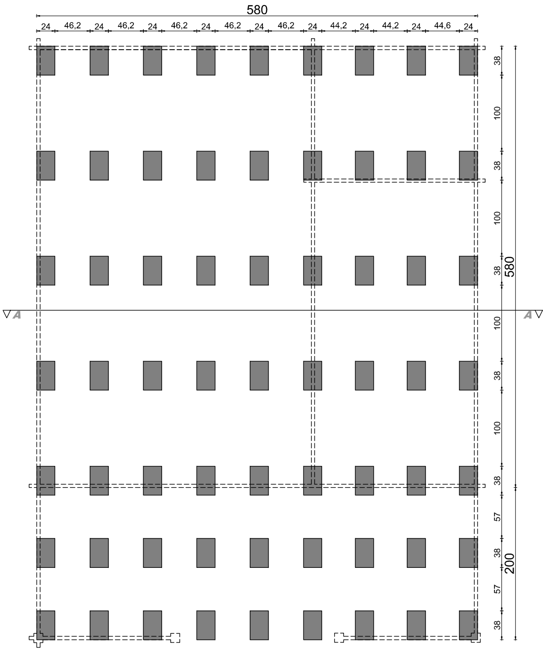
rzut fundamentów
