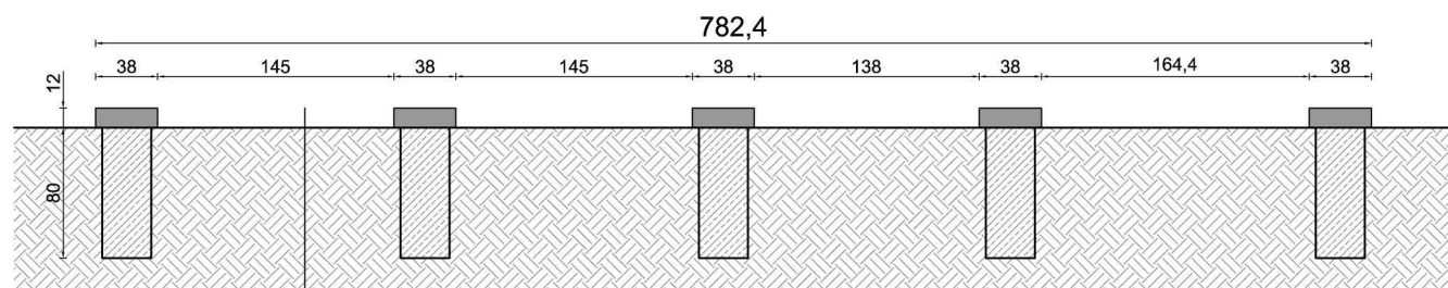
przekrój A-A
