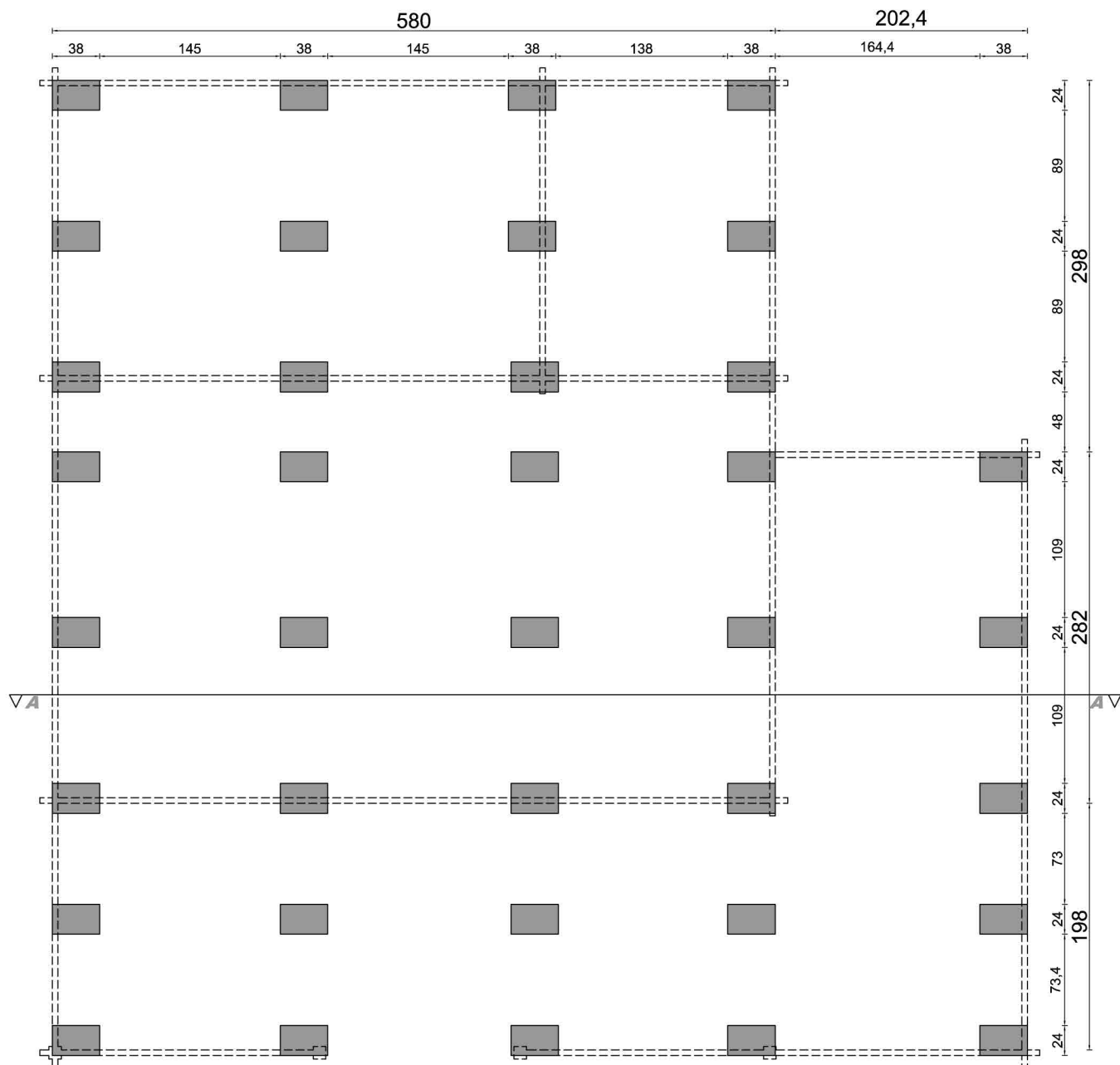
rzut fundamentów
