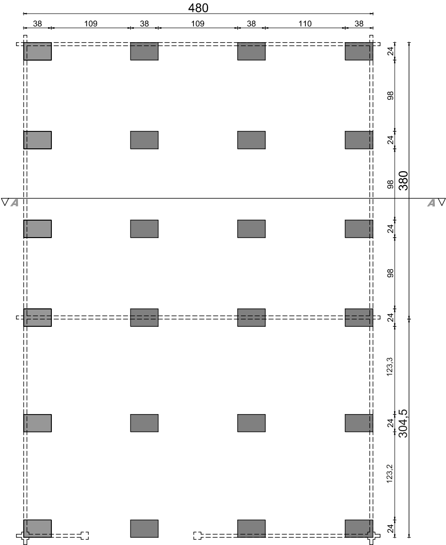
rzut fundamentów
