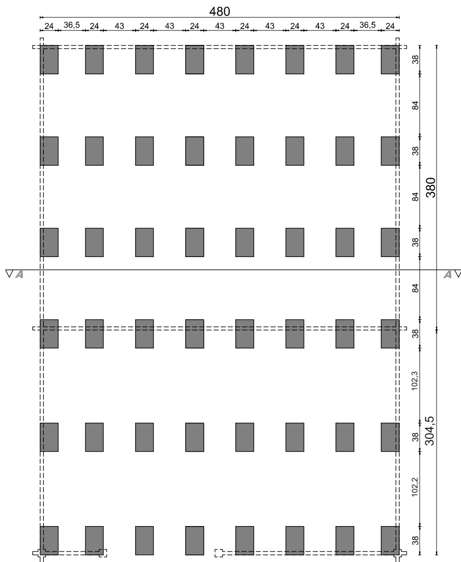
rzut fundamentów
