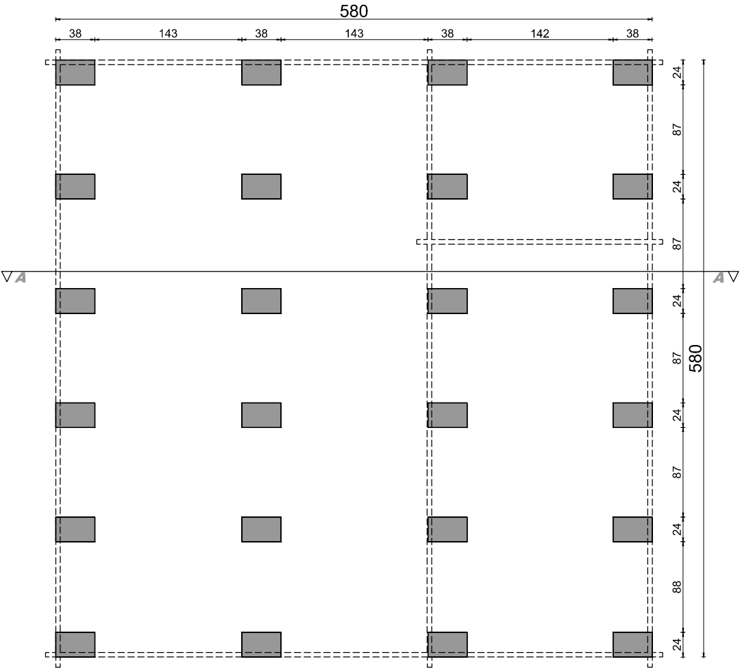
rzut fundamentów
