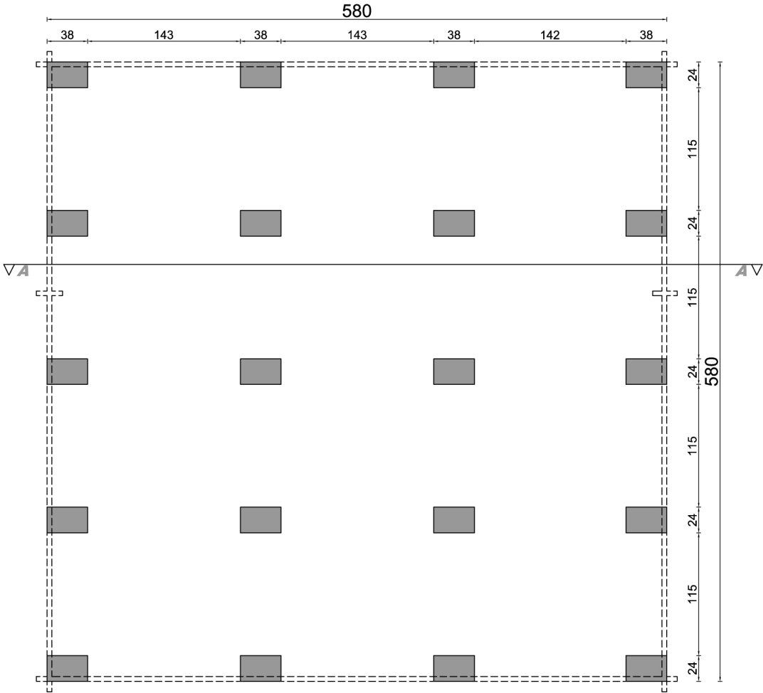
rzut fundamentów
