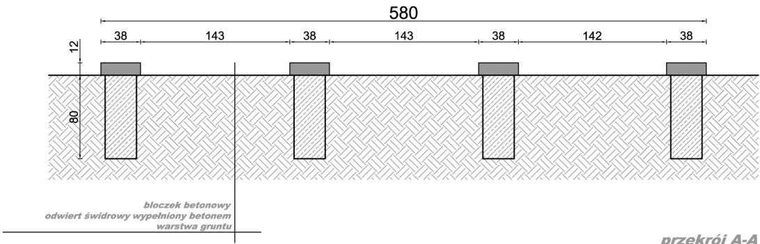
przekrój A-A
