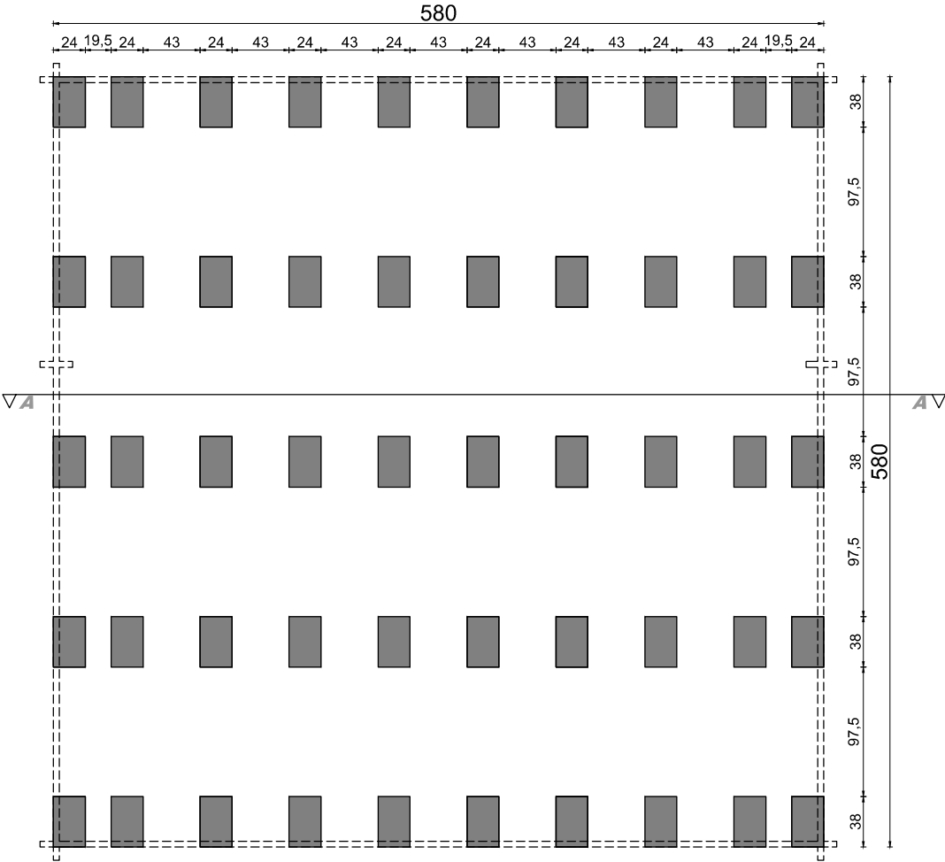
rzut fundamentów
