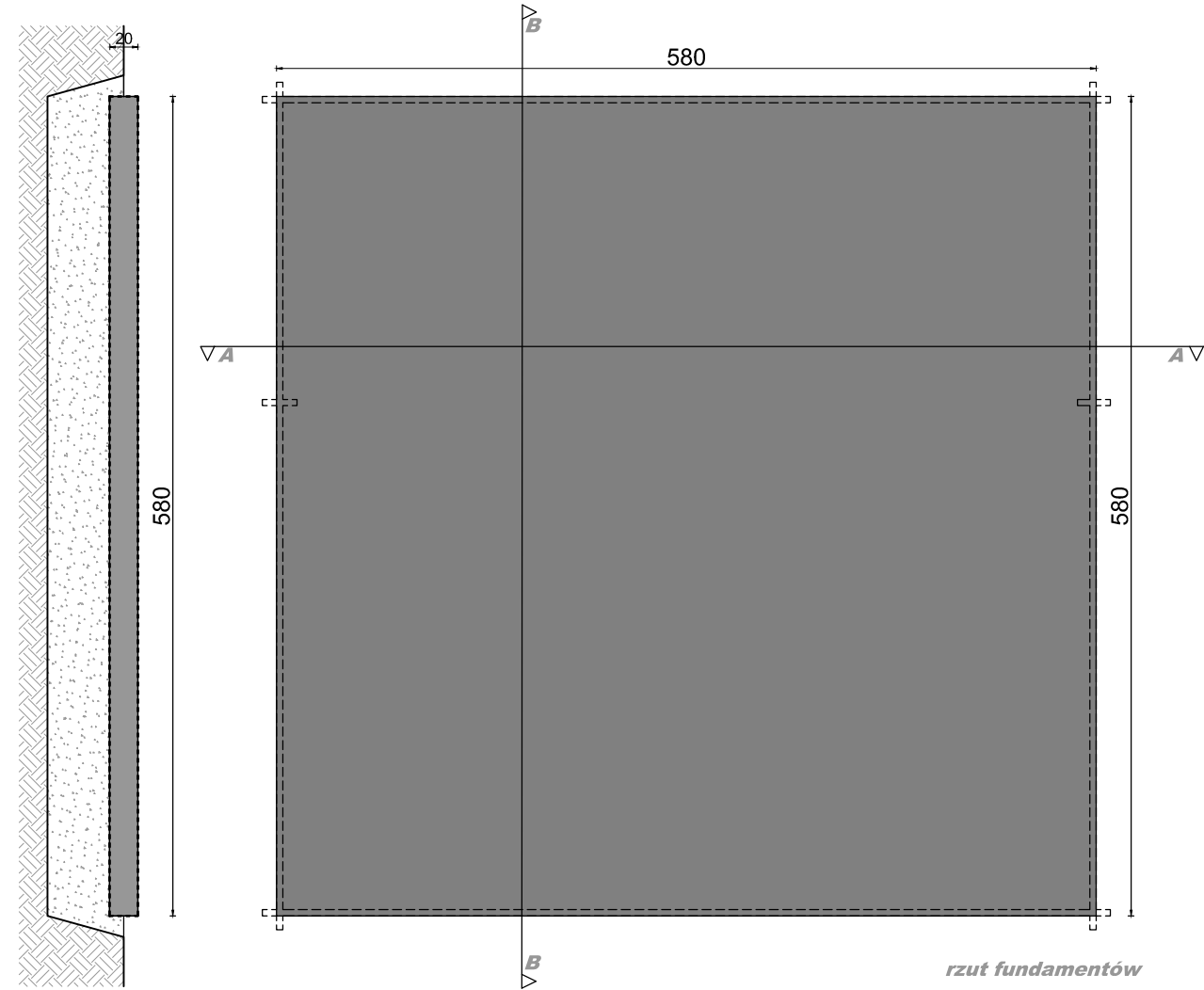
przekrój B-B
