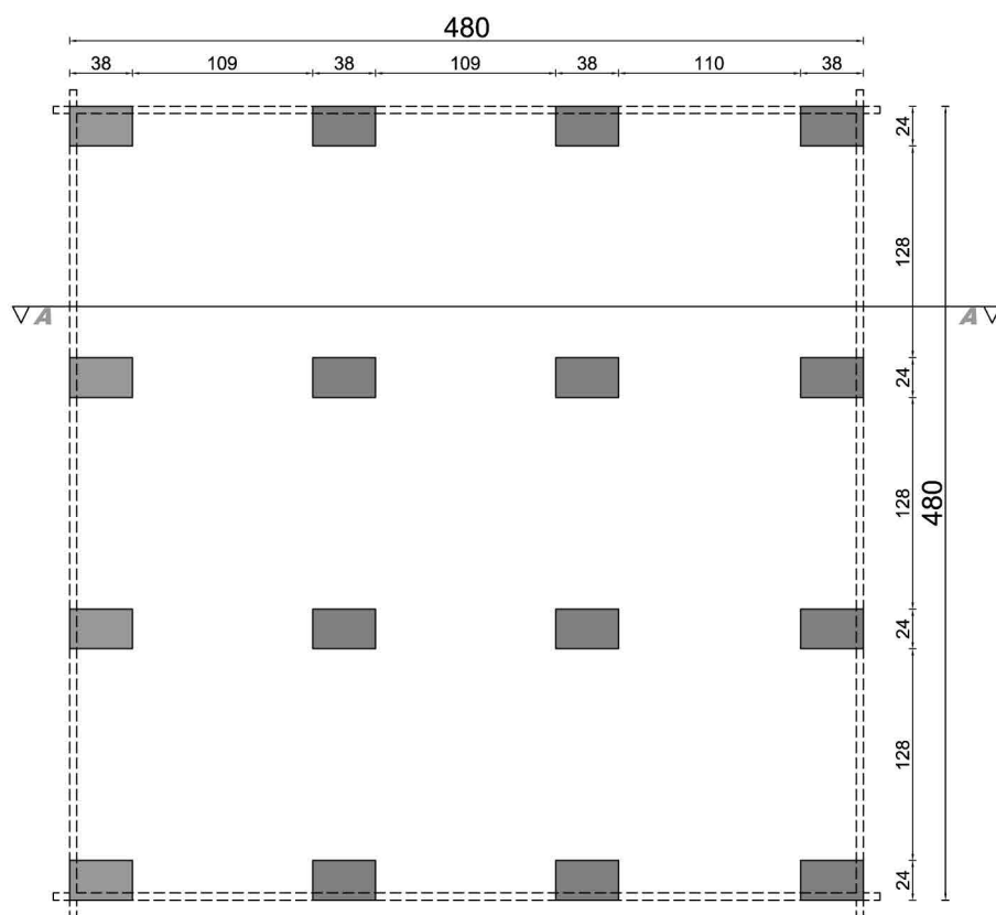
rzut fundamentów
