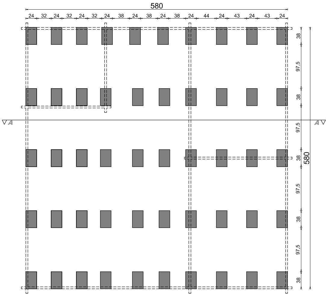
rzut fundamentów
