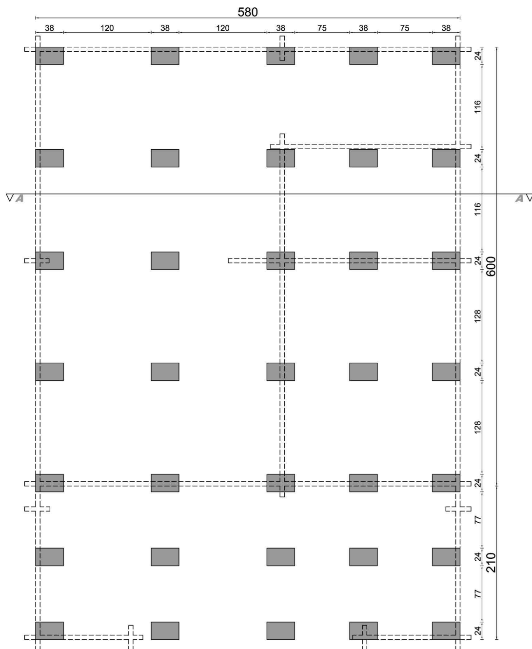
rzut fundamentów
