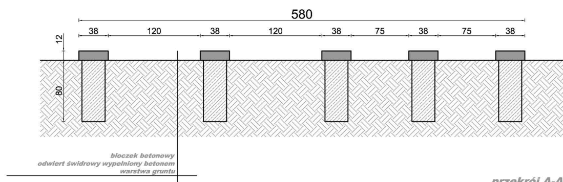
przekrój A-A
