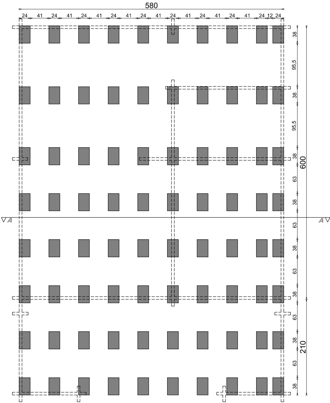
rzut fundamentów
