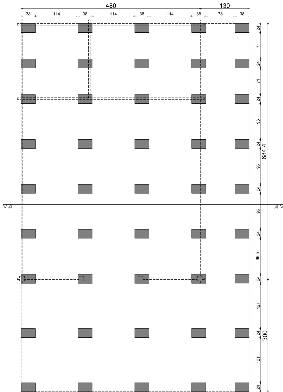
rzut fundamentów
