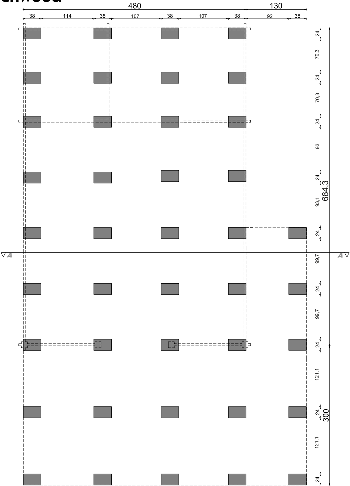
rzut fundamentów
