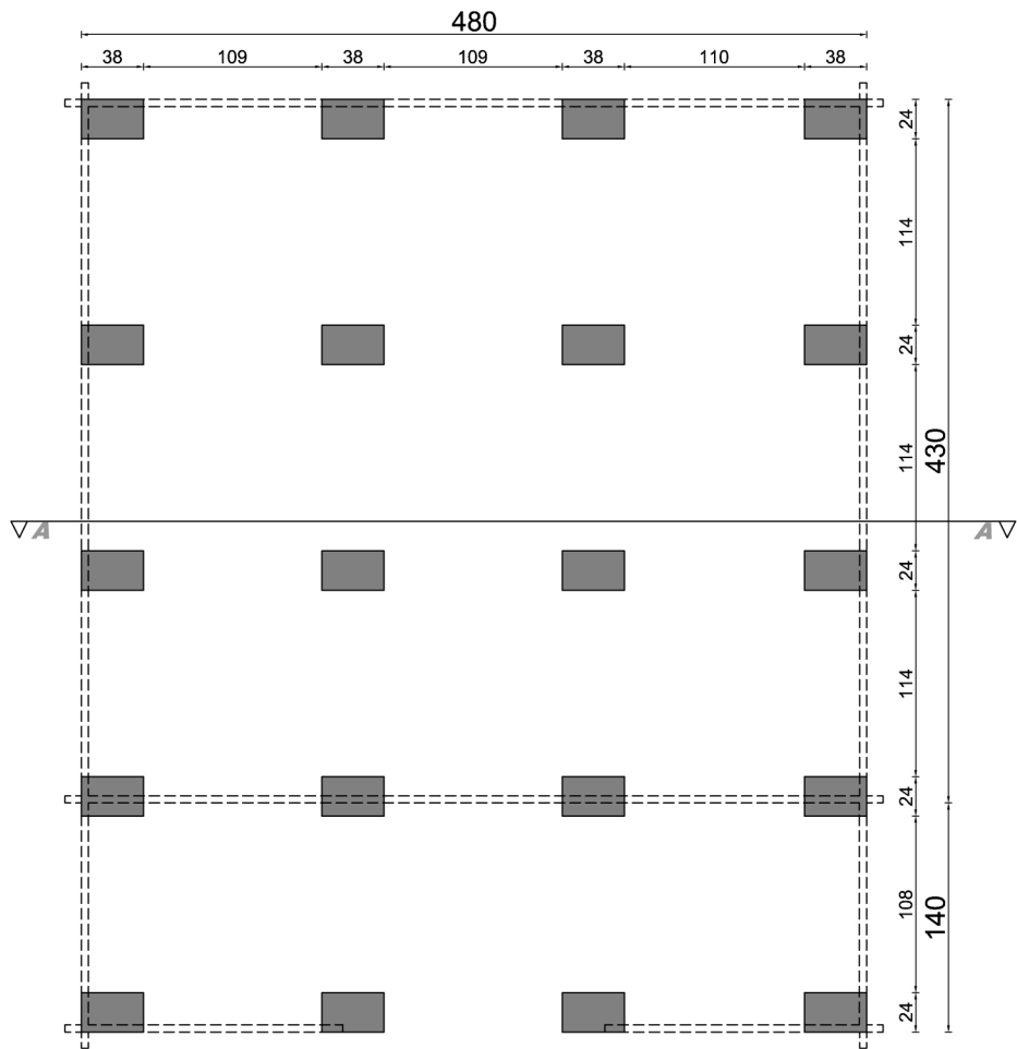
rzut fundamentów
