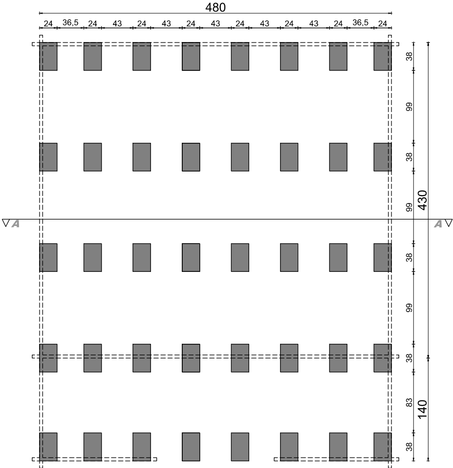
rzut fundamentów
