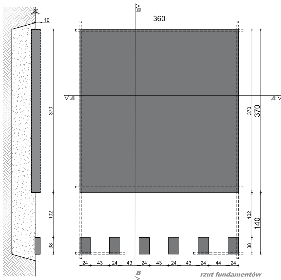
przekrój B-B
