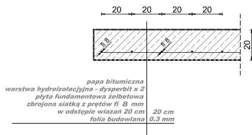
detal zbrojenia płyty fundamentowej
