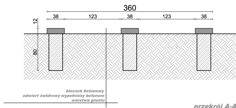
przekrój A-A
