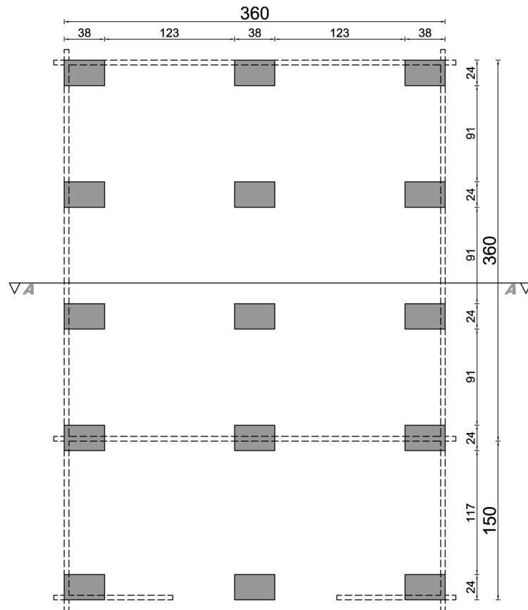
rzut fundamentów
