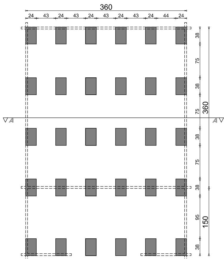
rzut fundamentów
