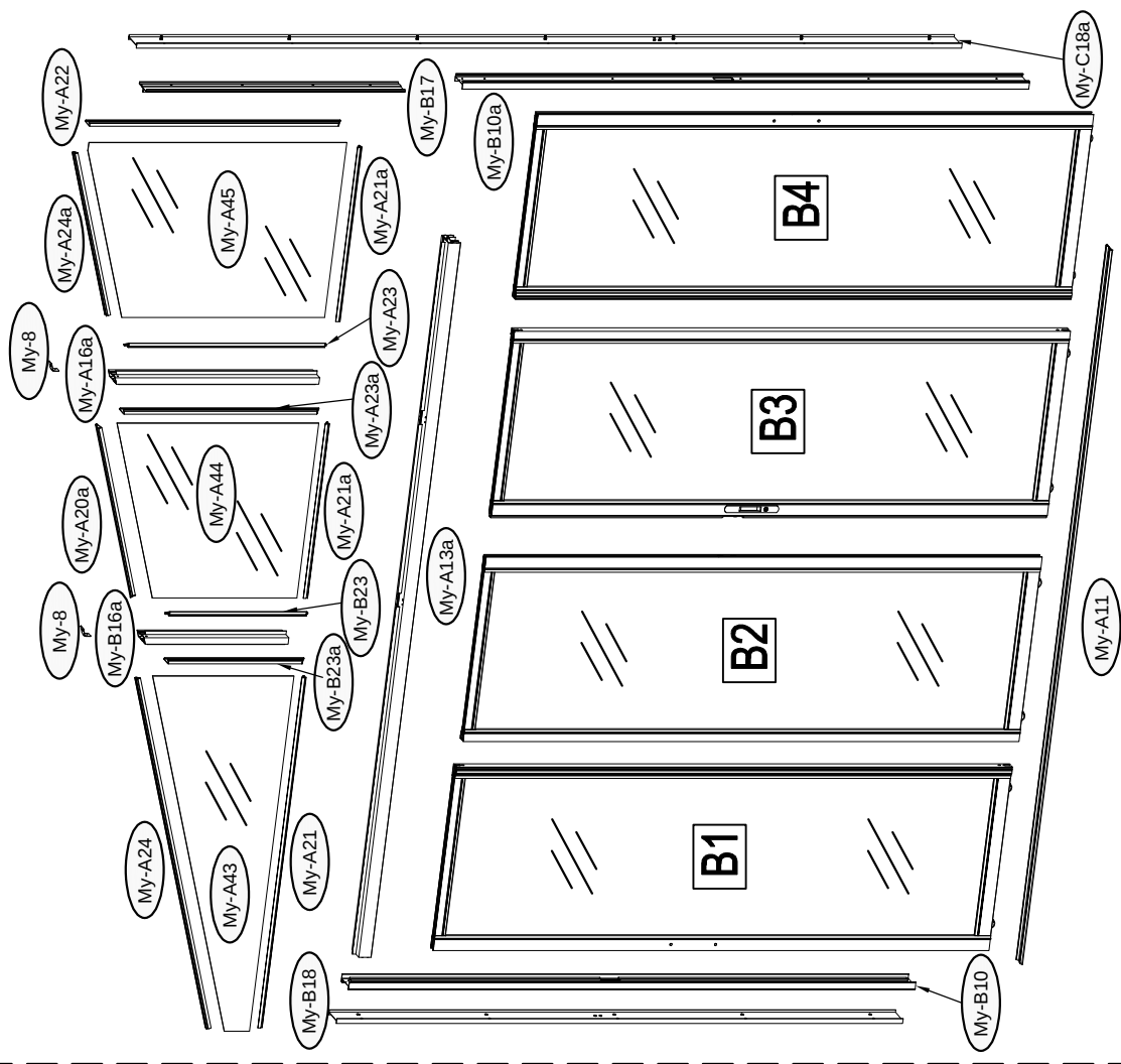
Prawa ściana i drzwi/Right wall & door
